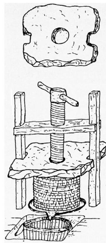
Esquema de funcionament d'un trull o premsa medieval, segons Albert Benet.
