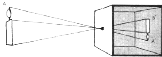
Esquema de funcionament de la càmera estenopecica
