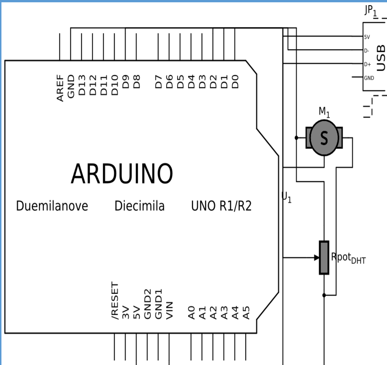
ESQUEMA ELÈCTRIC
