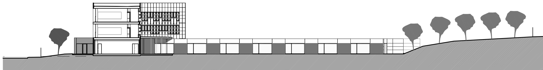
ALÇAT OEST 1 - INTERIOR
