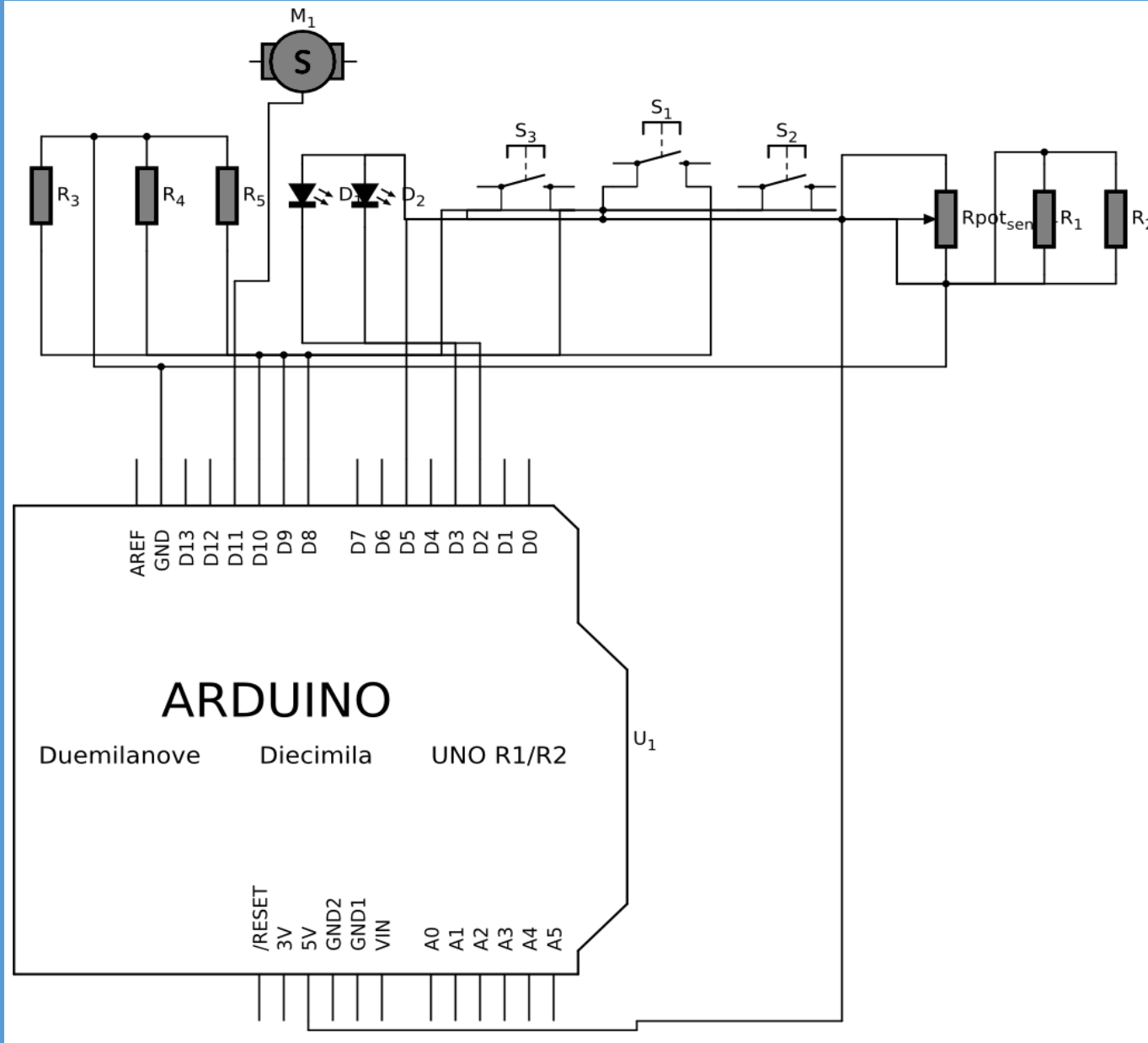
ESQUEMA ELÈCTRIC
