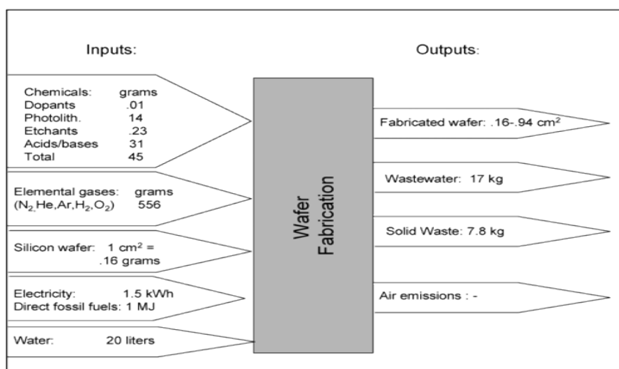
Ilustración 2: Material y energías necesarios para fabricar 1 cm 2 (0.16 gramos) de microcircuitos sobre una oblea de silicio. Sería el equivalente, por ejemplo, de un chip de memoria DRAM de 20 Mbytes [ERI3].
