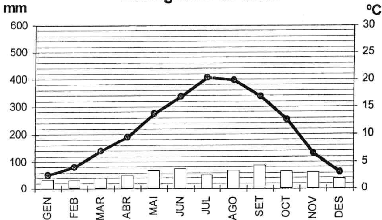
Climograma de Moià
