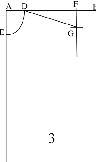
Figura.3 A-F=1/2 ample davant F-G=5 cm. baixada d'espatlla D-G=llarg d'espatlla
