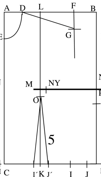
Figura.5 I'-J' s'uneixen en O N-P= profunditat pinça costat
