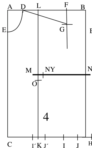
Figura.4 C-H=1/4 contorn de malucs C-I= 1/4 contorn de cintura 1/2 (I-H)= J 1/2 (C-J)= K I-J es trasllada a ambdós costats de K= I'-J' K-L= línia centre davant L-M= baixada de pit M-N= línia pinça pit M-NY= 2 cm. separació pinça costat M-O= 2cm. sepració pinça cintura
